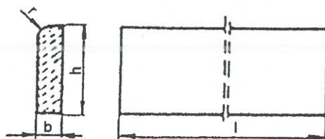
obrzeża chodnikowego
